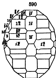
Vesuvius.
